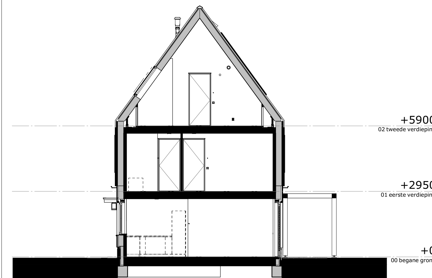
doorsnede A
