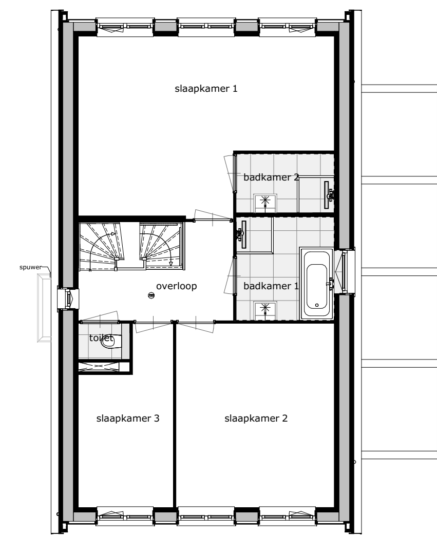
eerste verdieping
