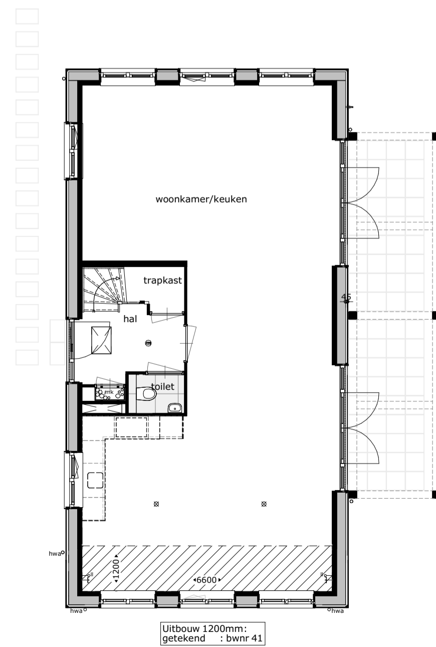
Uitbouw 1200mm: getekend : bwnr 41 begane grond: optie 00007
