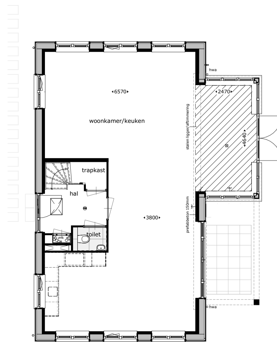
Erker zijgevel: getekend : bwnr 41 begane grond: optie 00042
