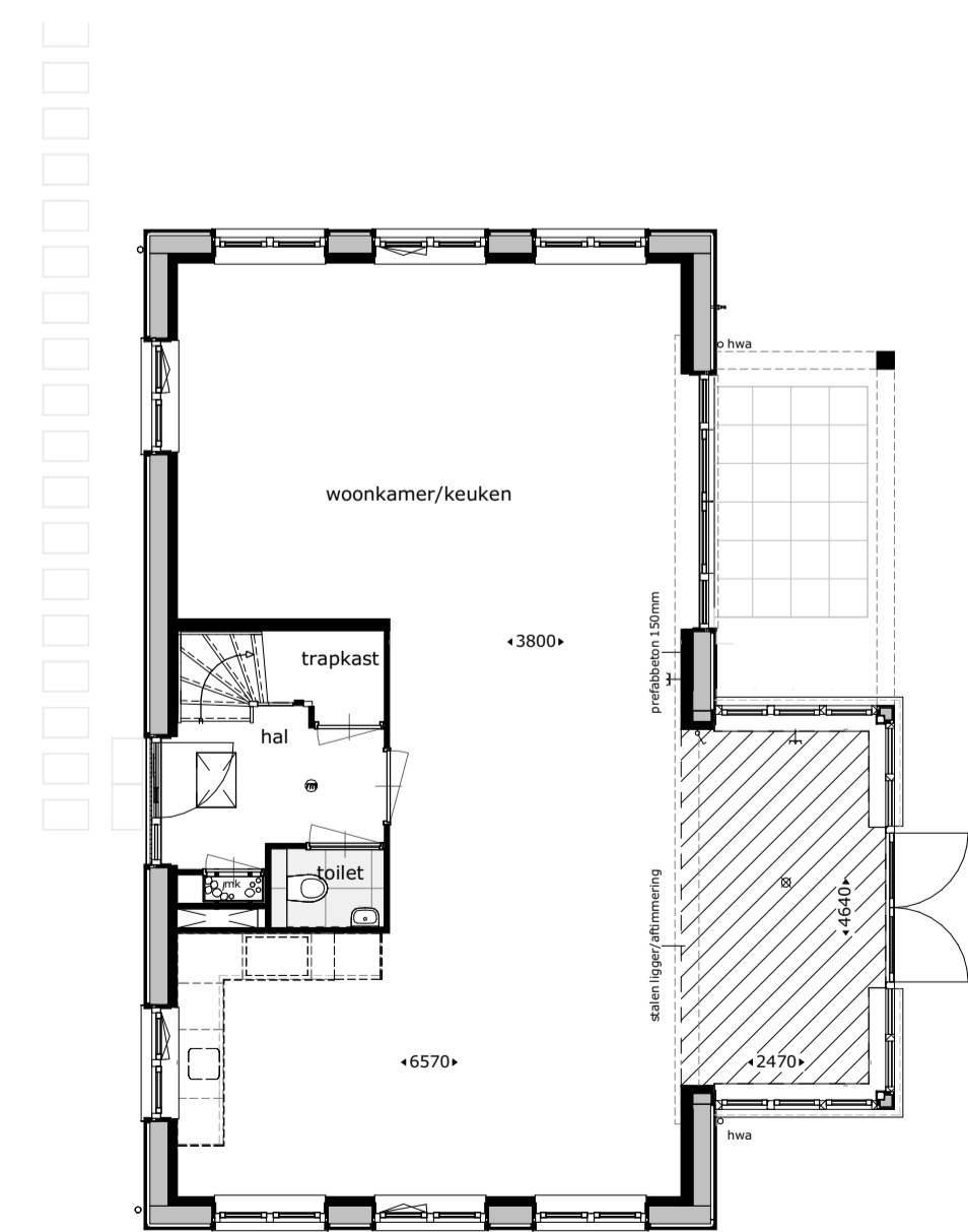
Erker zijgevel: getekend : bwnr 41 begane grond: optie 00041
