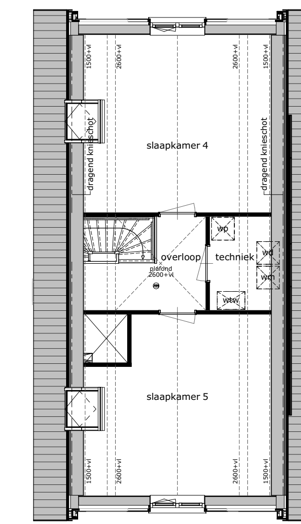
tweede verdieping
