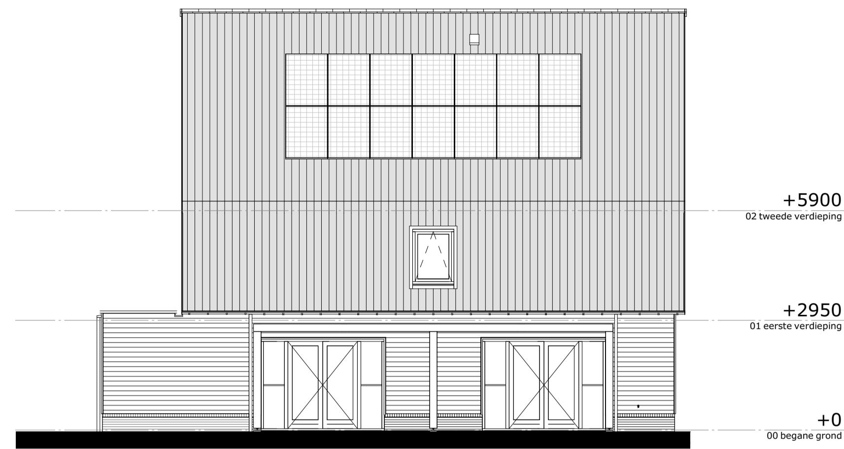
Uitbouw 2400mm: getekend : bwnr 41 achtergevel
