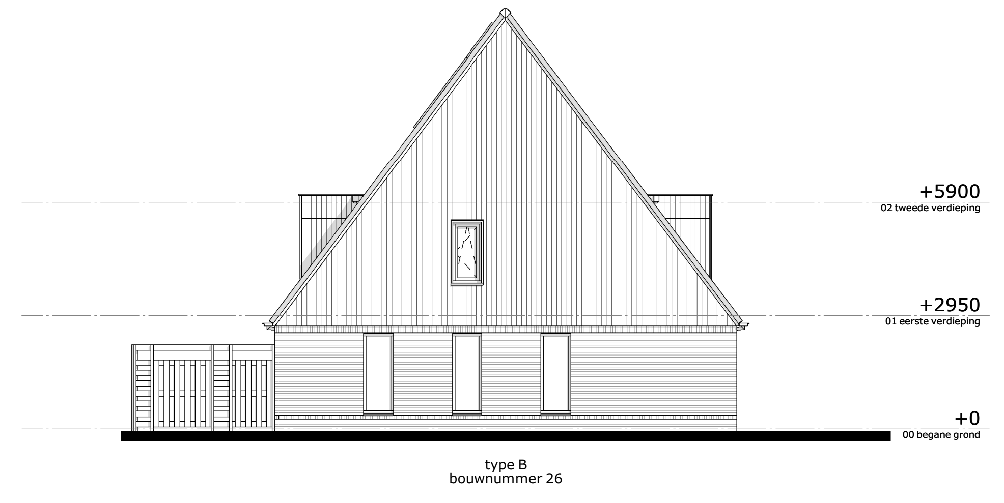
linker zijgevel
