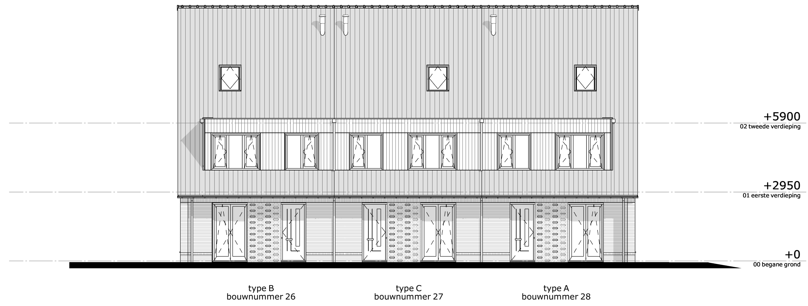
voorgevel
