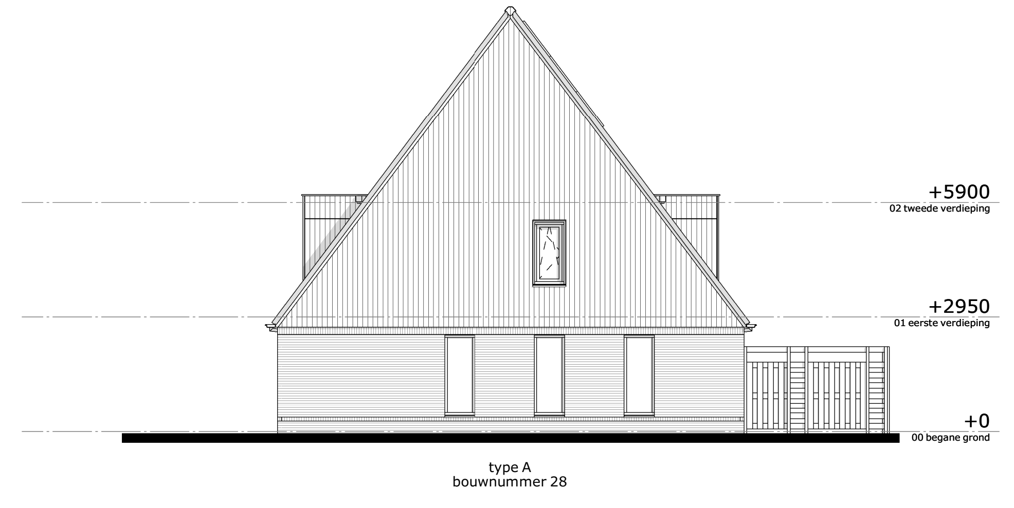
rechter zijgevel
