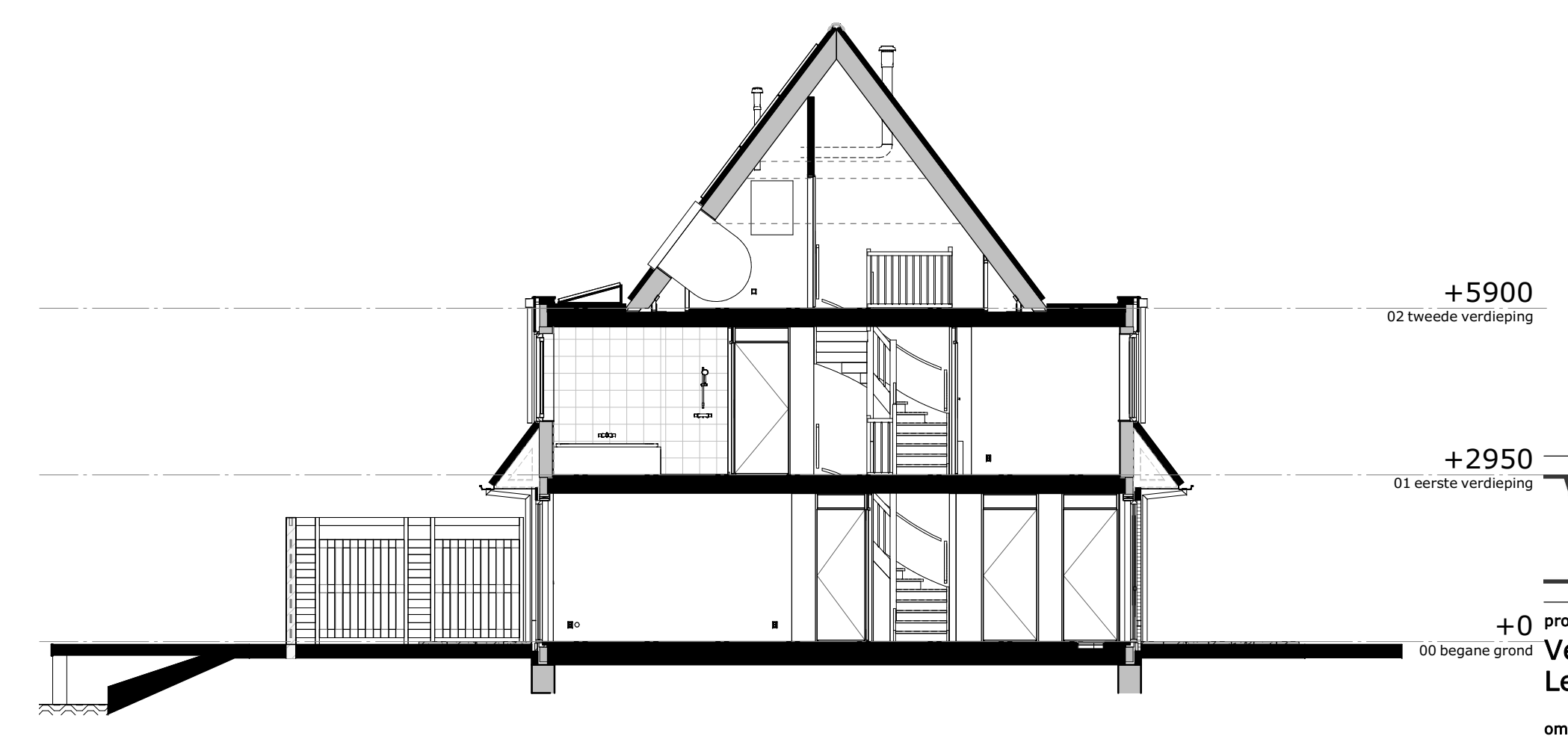
doorsnede A
