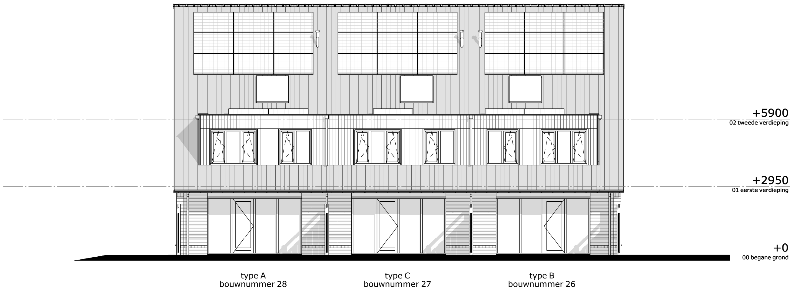
achtergevel
