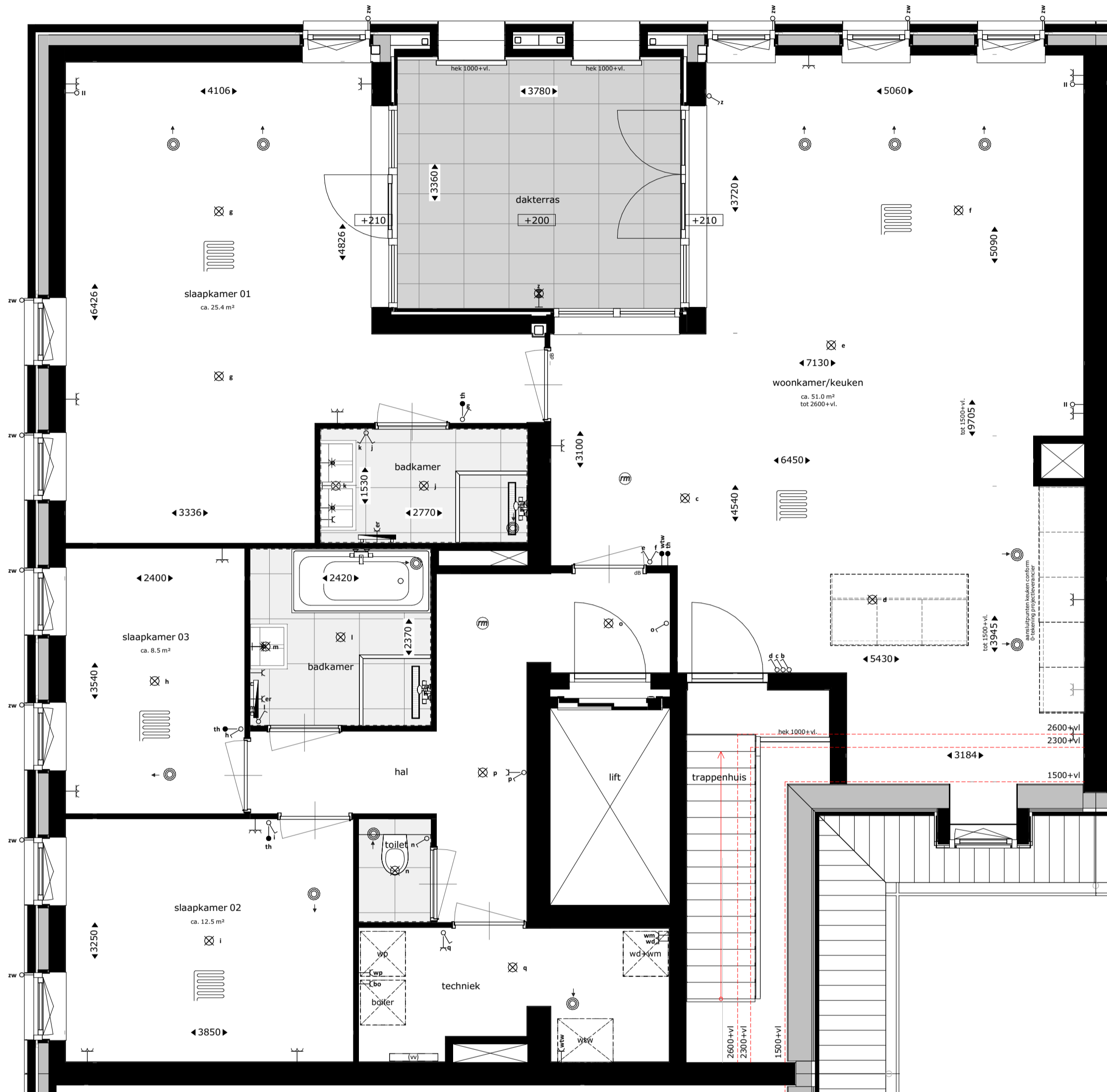
tweede verdieping
