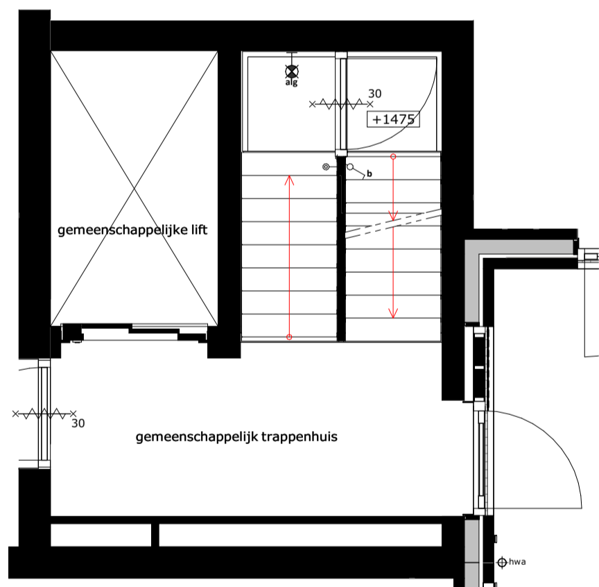
begane grond
