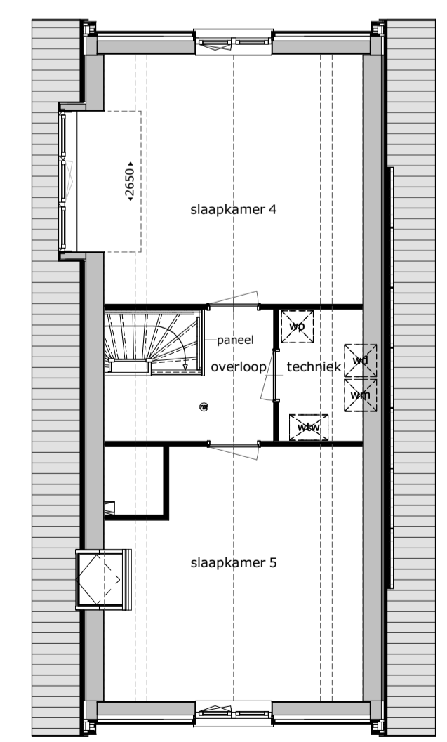
Dakkapel: getekend : bwnr 37 tweede verdieping: optie 30223
