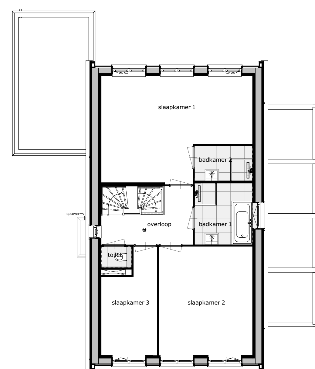
eerste verdieping
