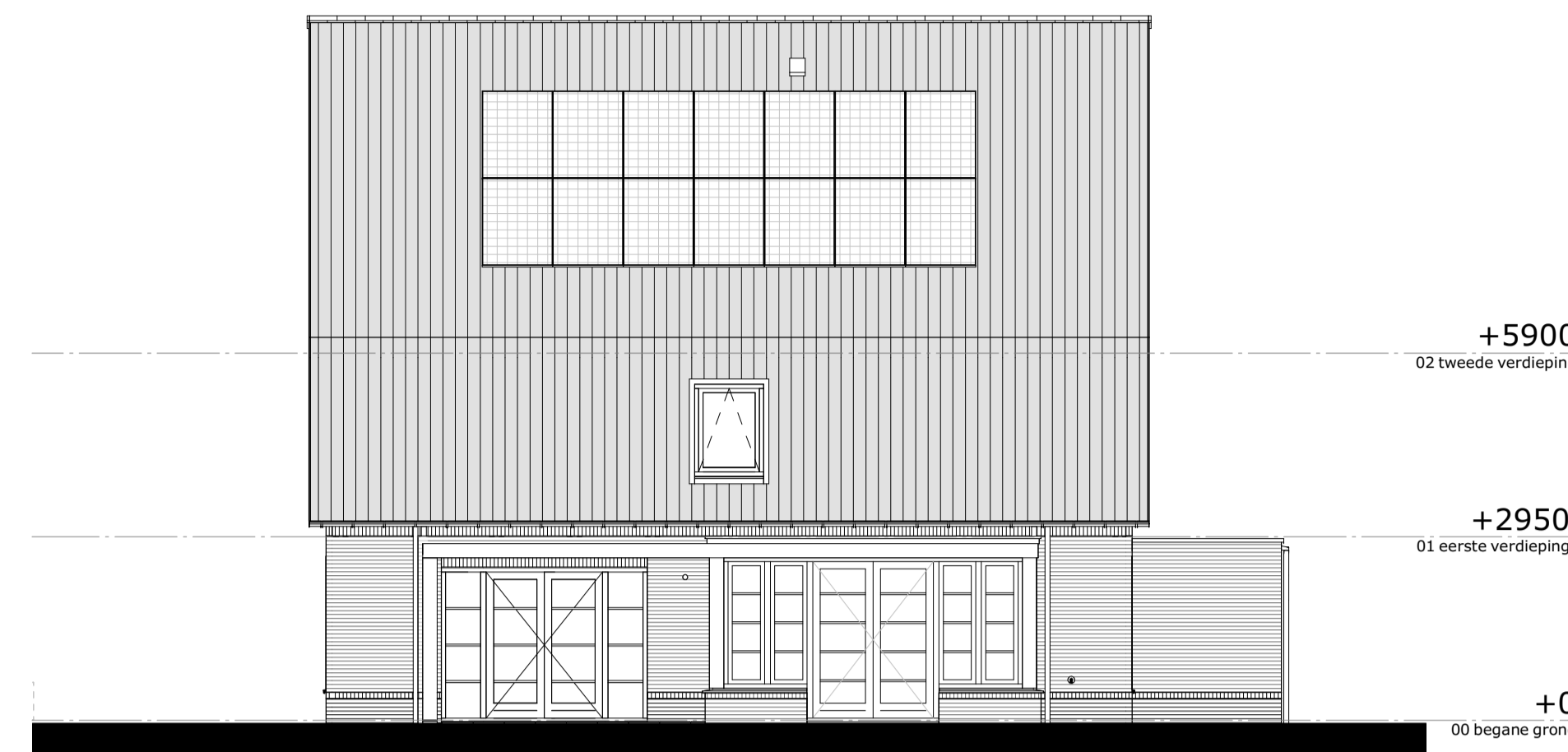
Erker zijgevel: getekend : bwnr 37 rechter zijgevel
