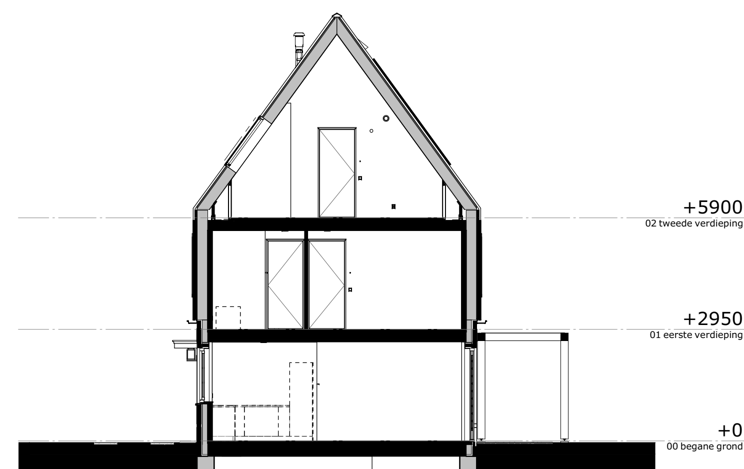
doorsnede A
