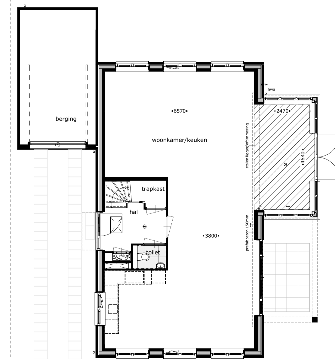
Erker zijgevel: getekend : bwnr 37 begane grond: optie 00042
