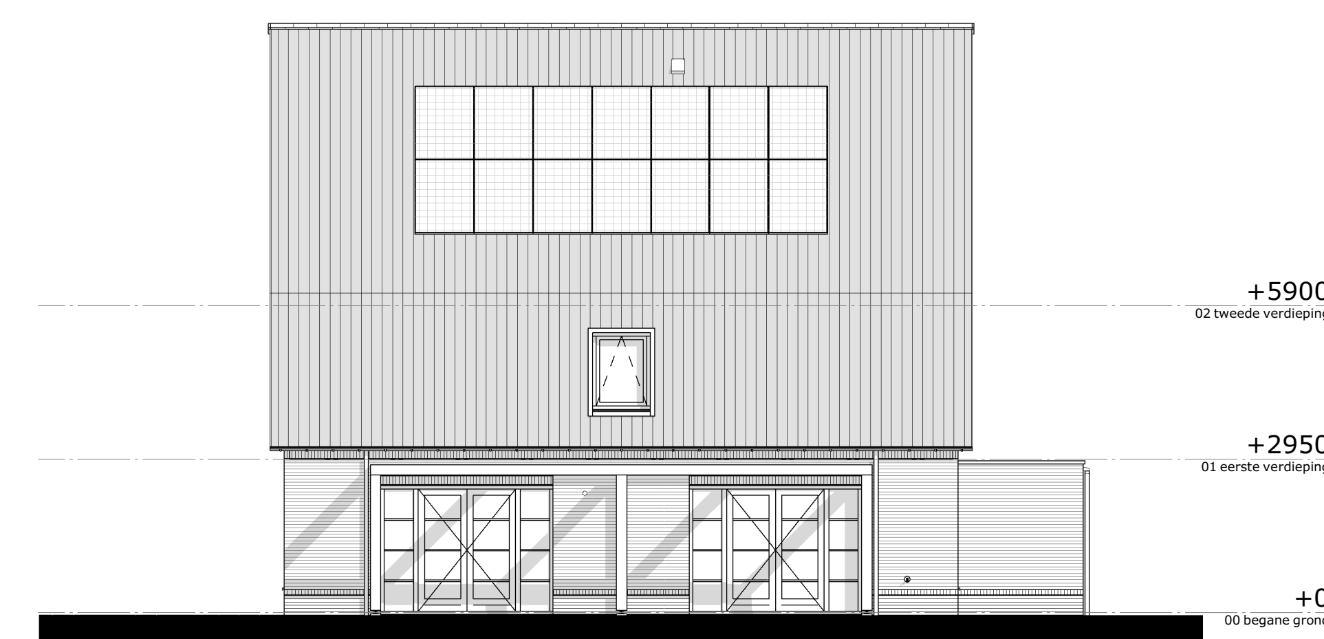
rechter zijgevel
