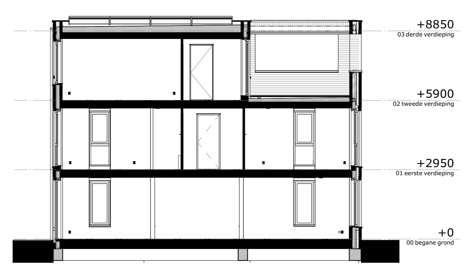
doorsnede B
