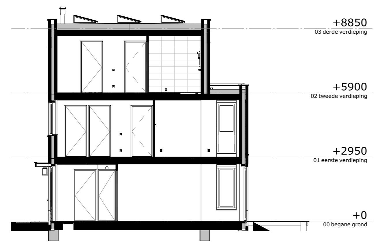
doorsnede A
