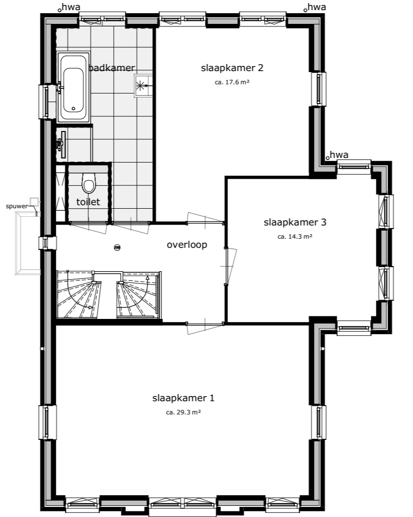
eerste verdieping
