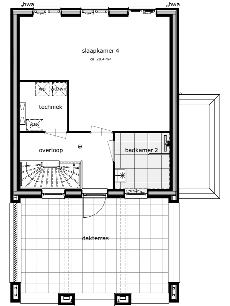
tweede verdieping
