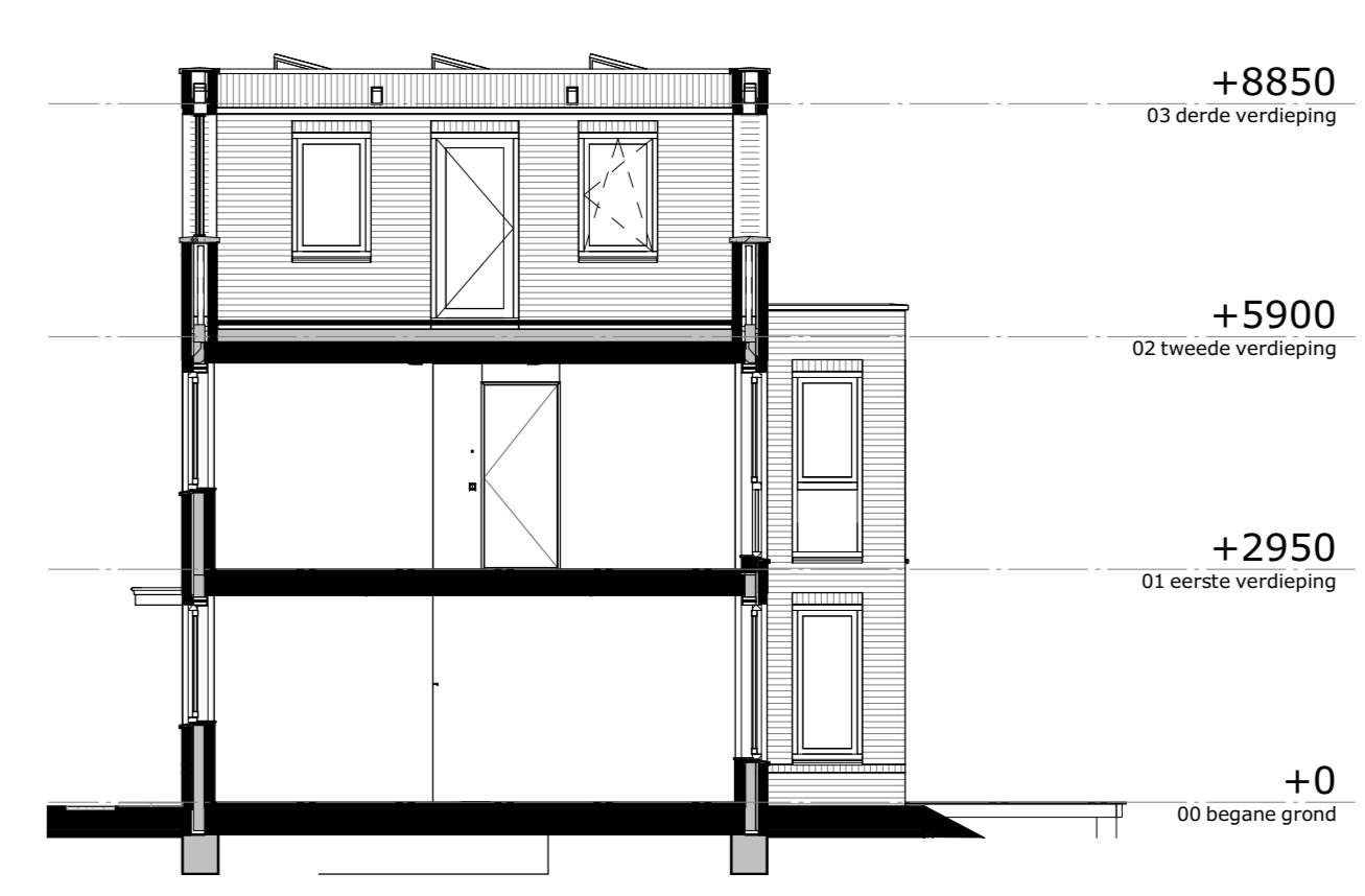
doorsnede C
