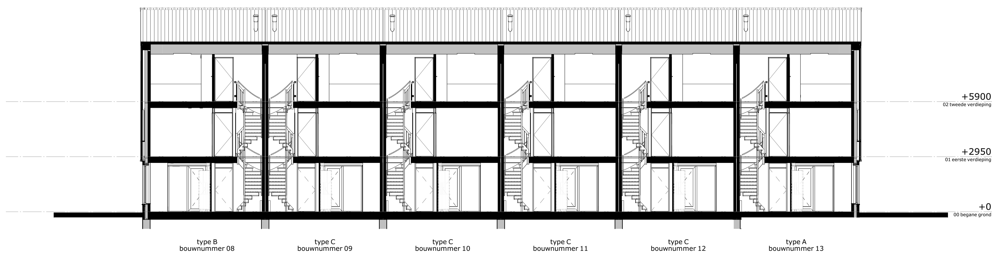
doorsnede B
