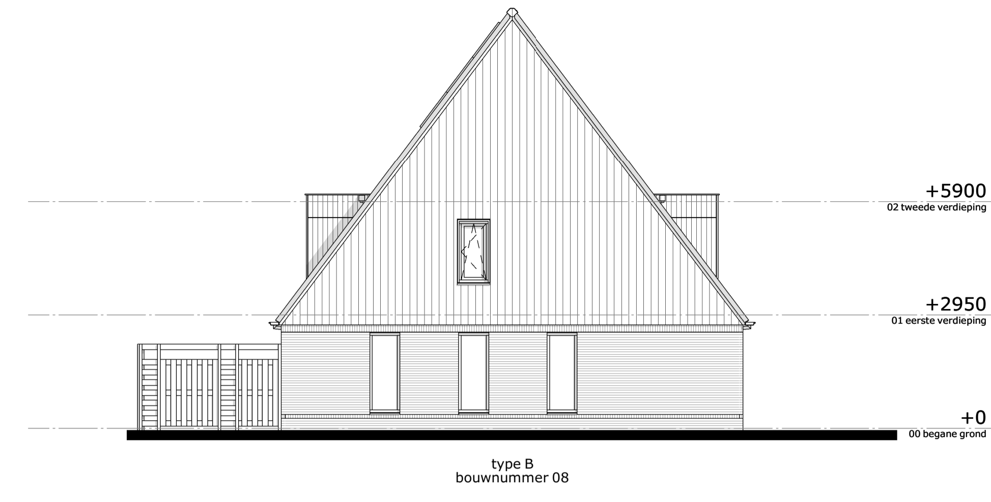
linker zijgevel
