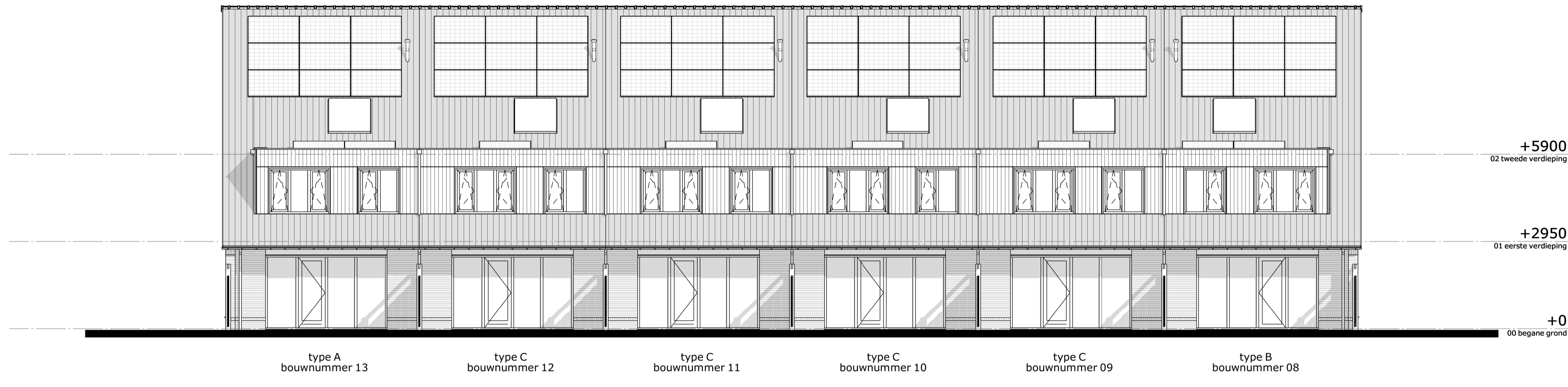
achtergevel
