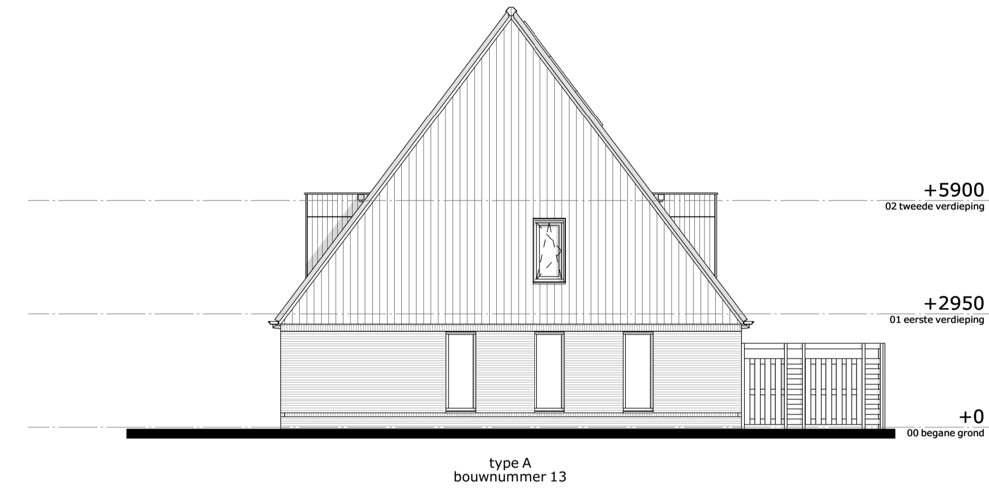
rechter zijgevel
