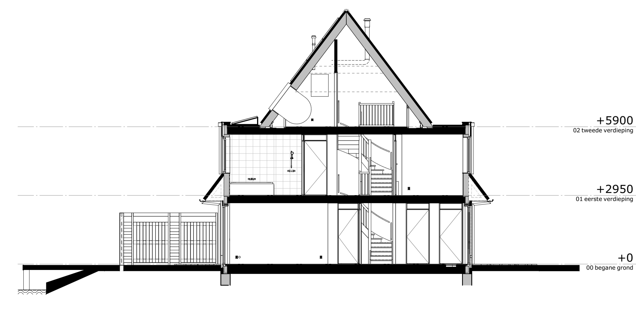
doorsnede A
