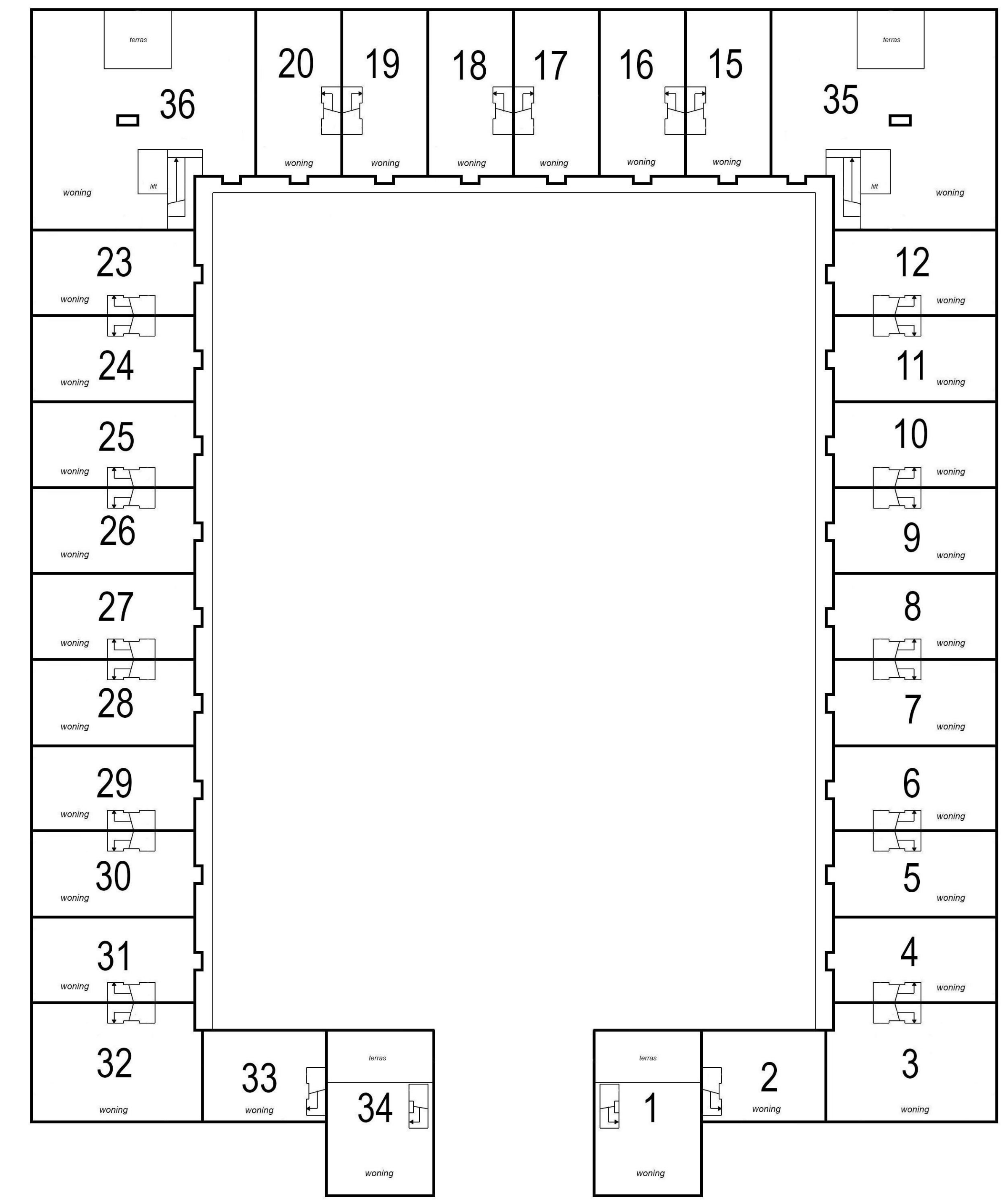
2e Verdieping 1:200
